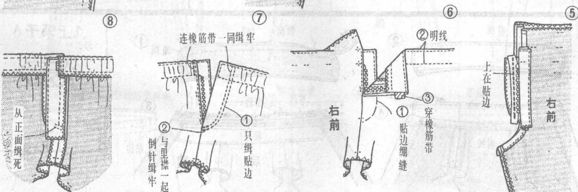
图⑥先合侧缝后做腰头
