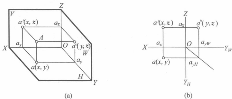
图 1-10 点的投影与坐标
