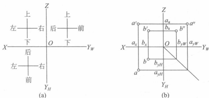
图 1-12 两点的相对位置
