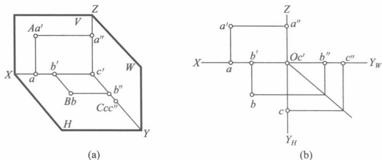
图 1-9 投影面、投影轴上的点的投影
