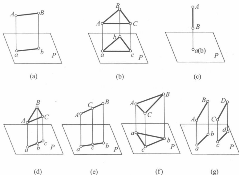
图 1-5 正投影的基本特性
