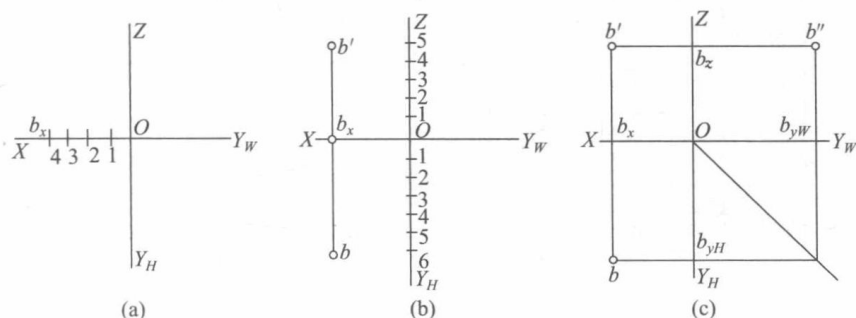
图 1-11 已知点的坐标，求点的三面投影
