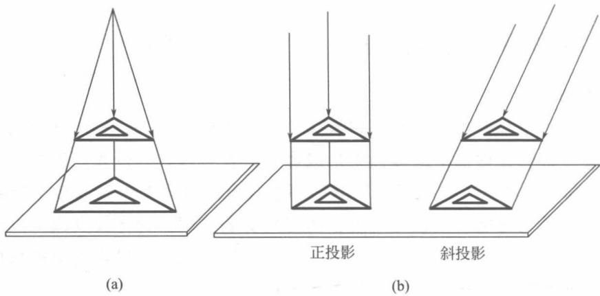
图 1-3 投影的分类 (a) 中心投影；(b) 平行投影
