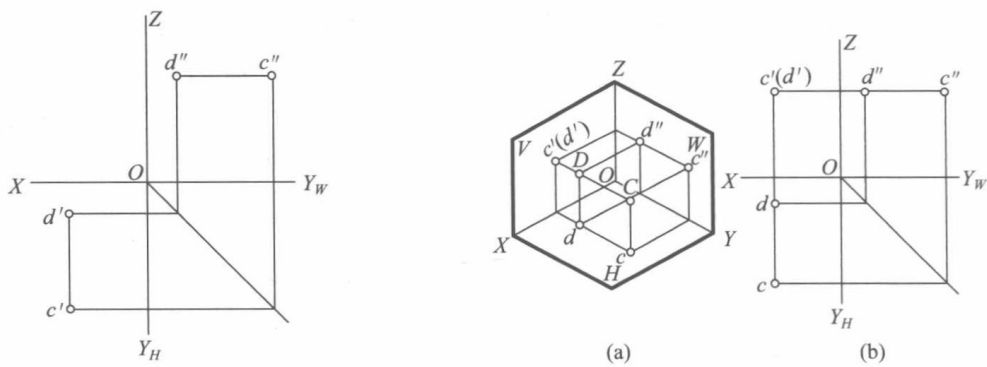
图 1-14 重影点的投影和可见性
