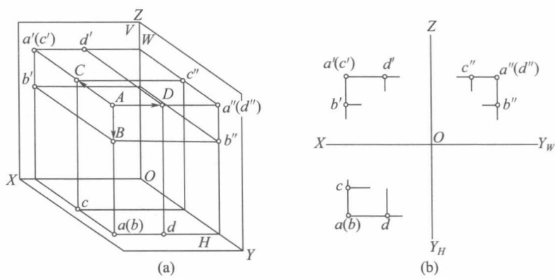
图 1-13 重影点的可见性 (a) 空间状况；(b) 投影图
