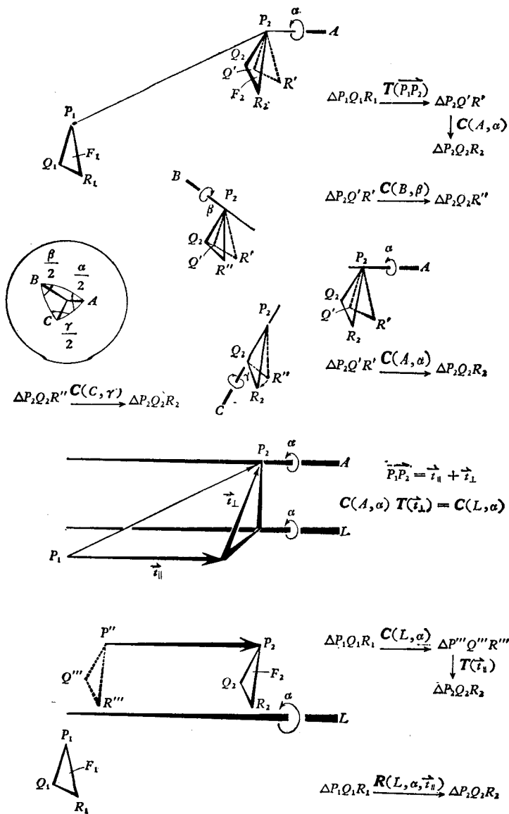
图 1.5 第一类重合操作和有关定理
