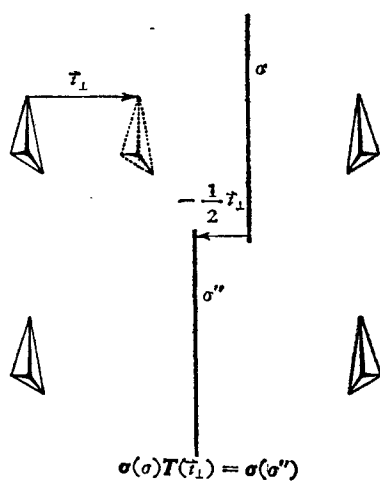
图 1.3 平移与反映的归并定理
