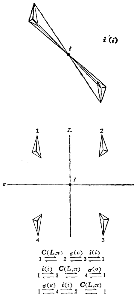
图 1.4 沟通反映和倒反的定理
