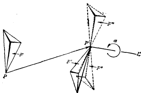
图 1-6 第二类重合操作和有关定理
