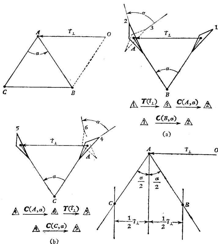
图 1·2 平移与旋转的归并定理
