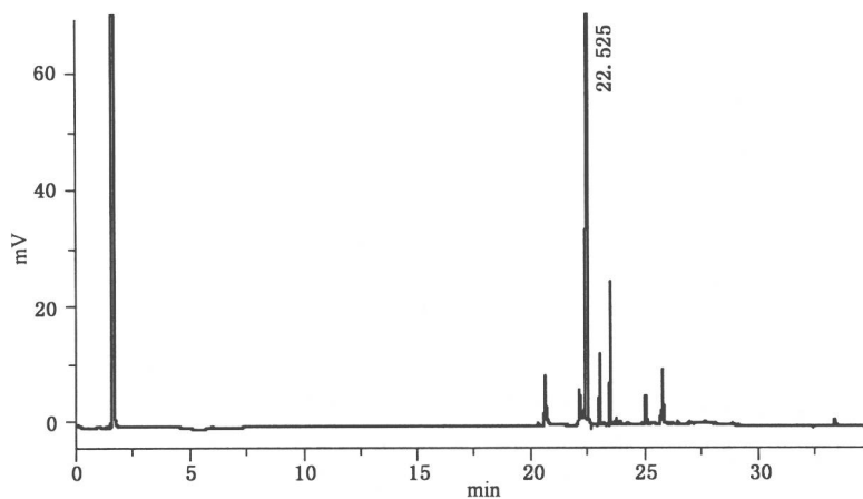
图 1 防老剂 4010NA 的色谱图
