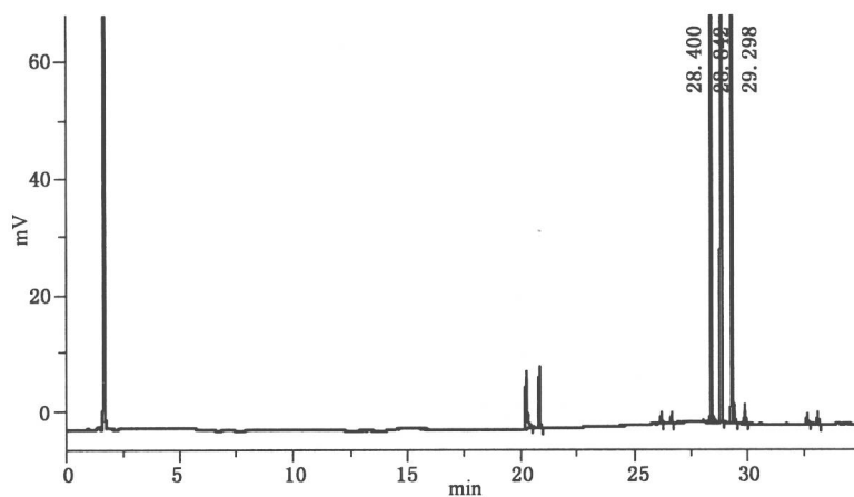
图 3 防老剂 3100 的色谱图
