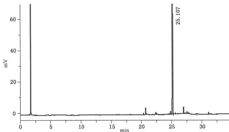
图 2 防老剂 4020 的色谱图
