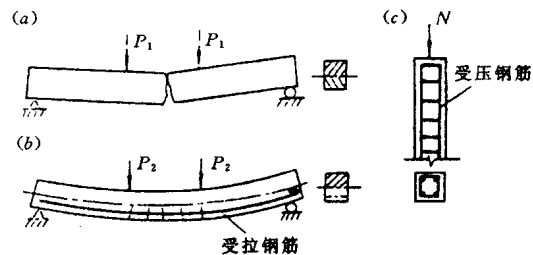
图 1-1 简支梁
