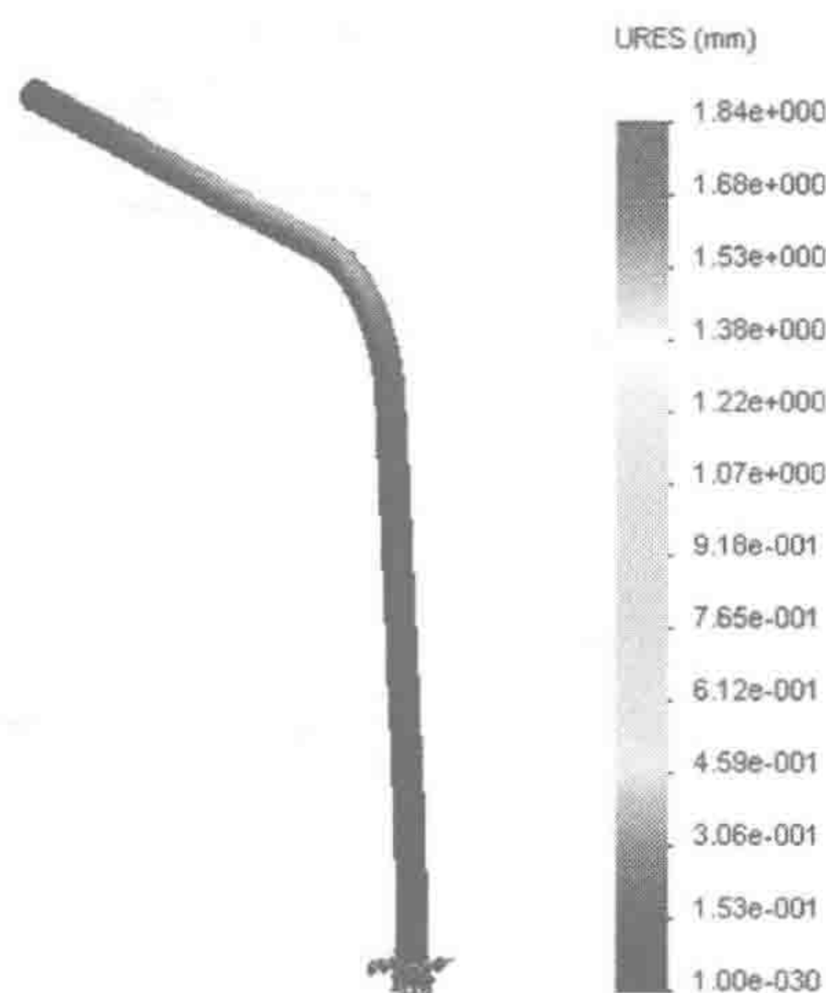
图 1-6 位移结果
