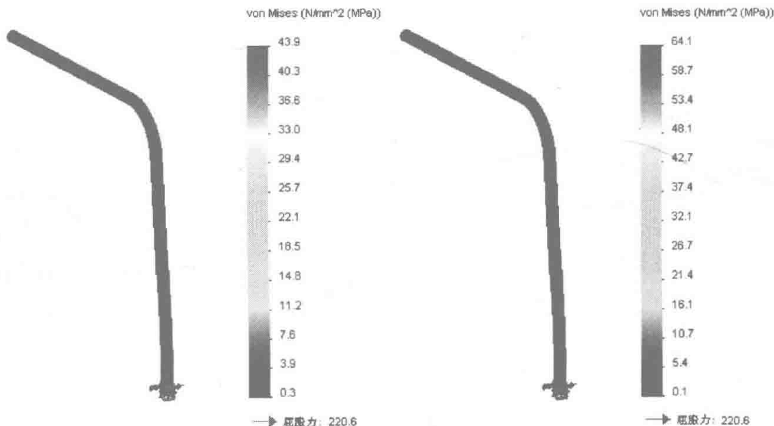
图 1-5 应力结果
