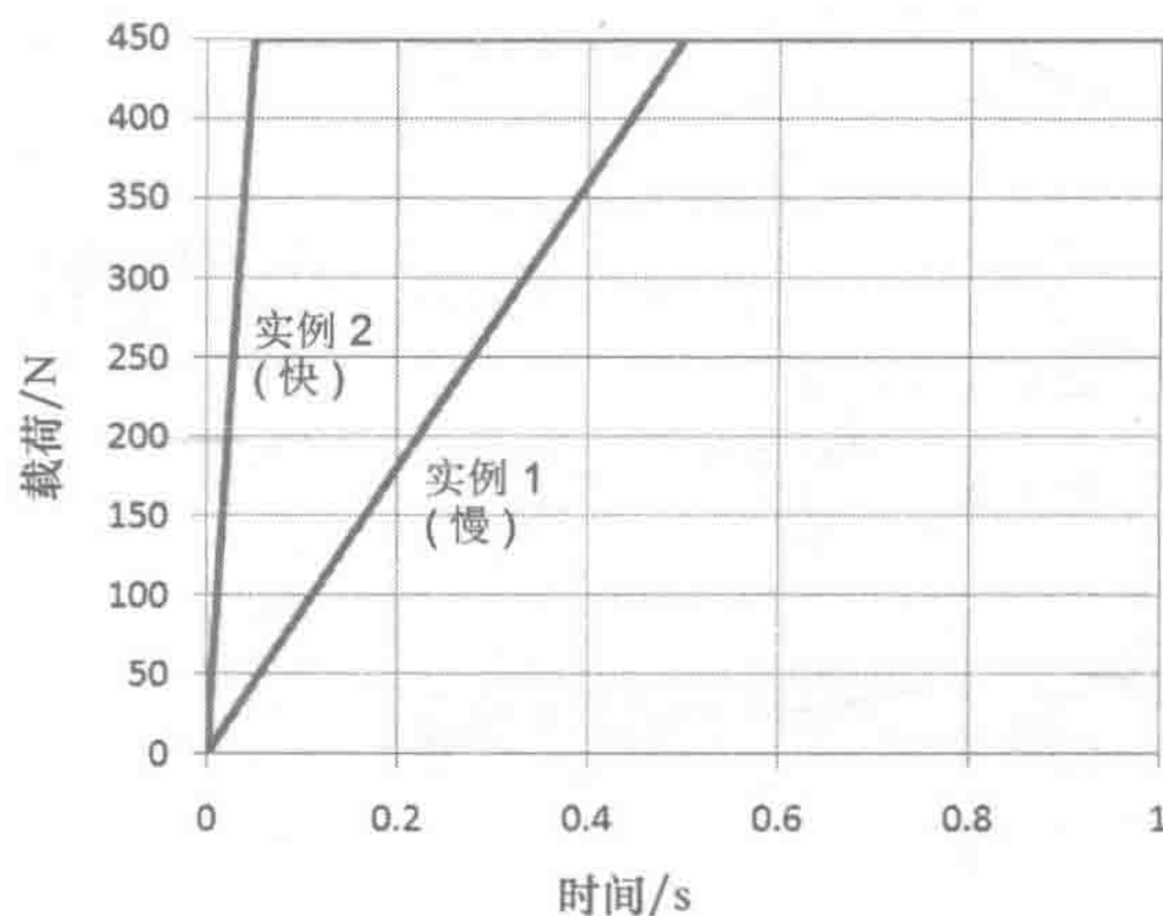
图 1-9 两种载荷的加载方式
