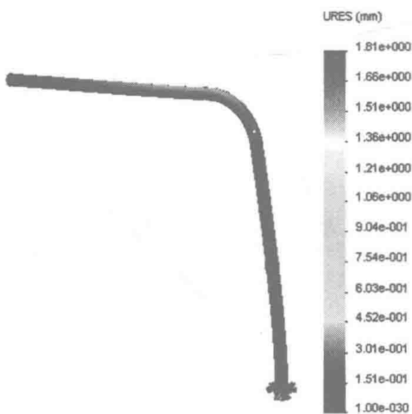
图 1-16 位移结果
