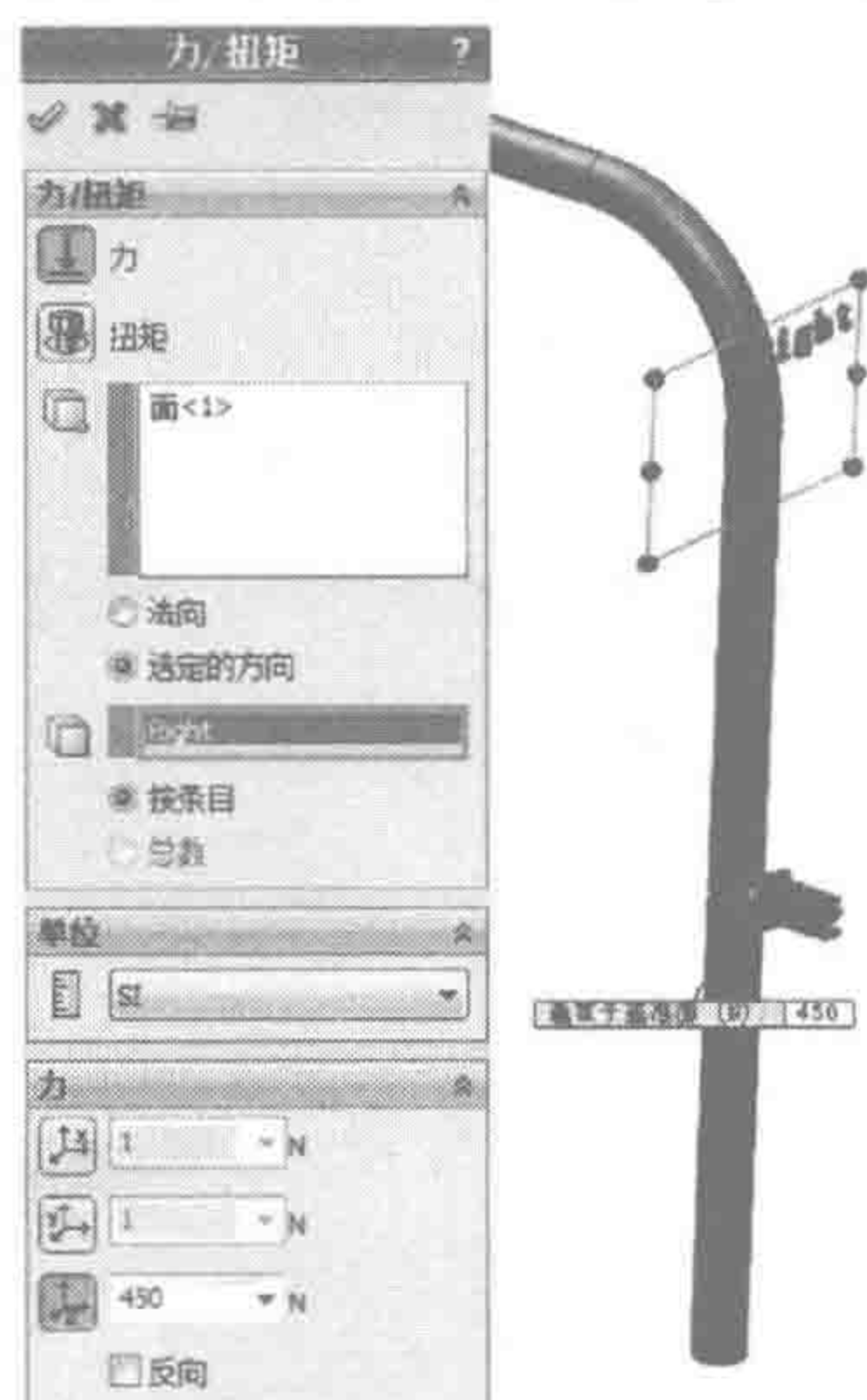
图 1-3 定义力
