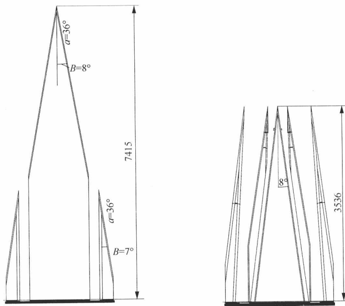
图 1.6 轧制 RD2 车轴的单楔与多楔模具
