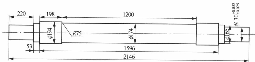
图 1.5 铁道车辆 RD2 轴
