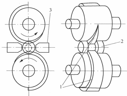
图 1.1 楔横轧工作原理图
