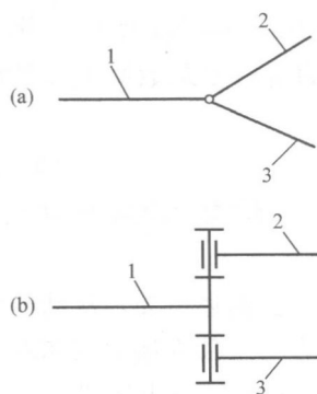
图 2-10 复合铰链
