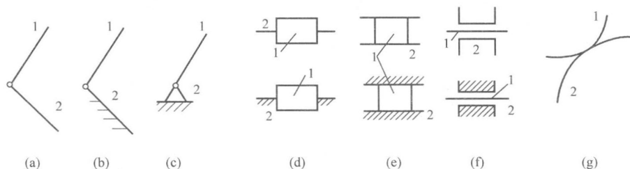
图 2-2 平面运动副的表示方法
