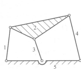
图 2-9 F=0 的构件组合
