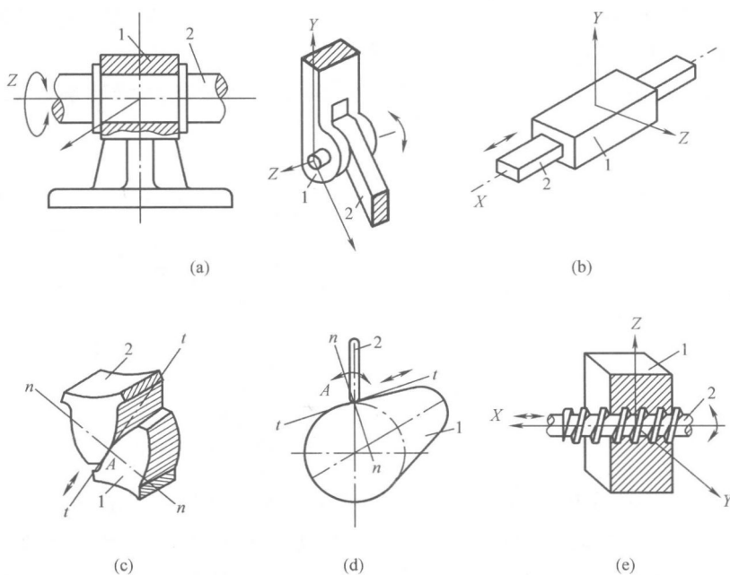
图 2-1 运动副
