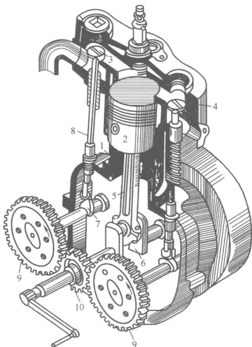
图1-1 内燃机
