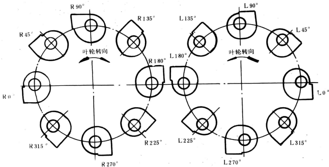
图 2 从防爆电动机端正视
