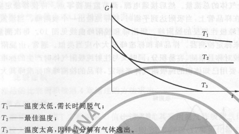
图 8 样品热重分析曲线
