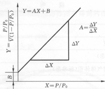
图 2 BET 图
