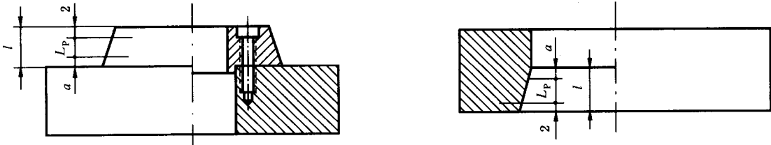
图 6 测量长度 L_P
