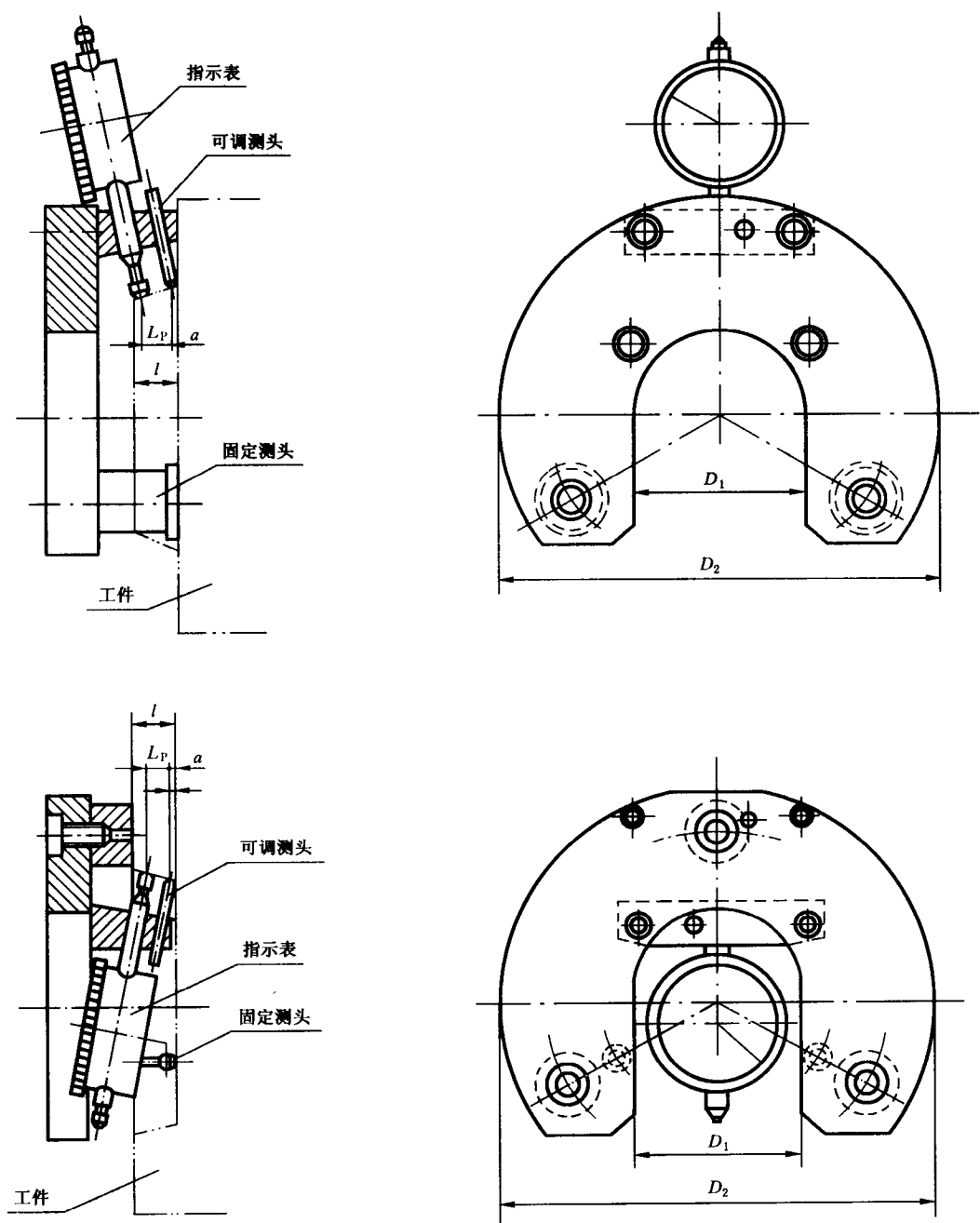
图 5 5 至 28 号 1/4 圆锥工作量规(指针式)的型式
