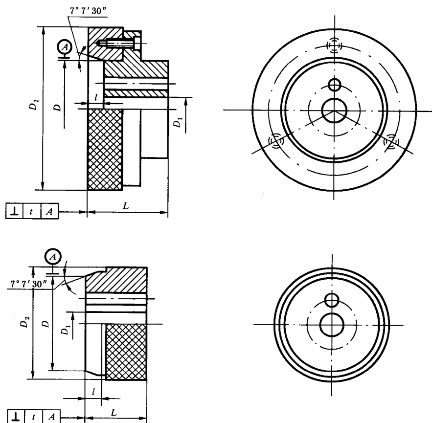
图 3 2 号 1/4 圆锥工作量规的类型
