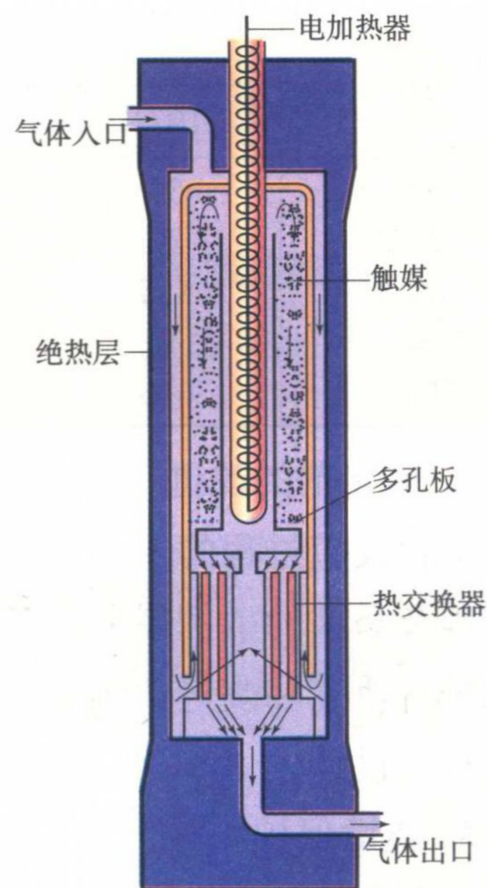
图1-9 合成塔内部构造示意图
