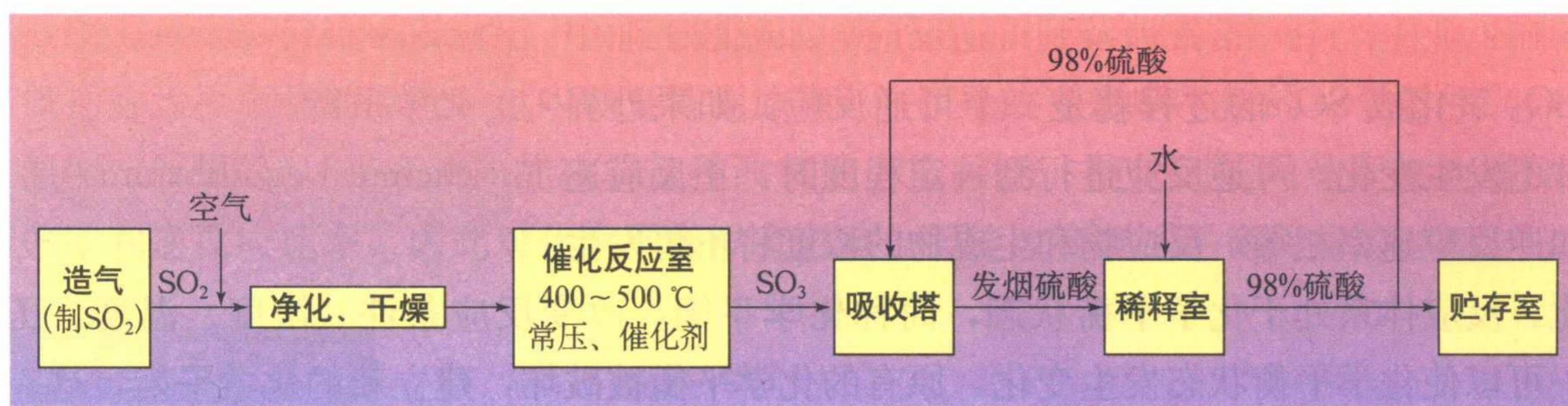
图 1-2 硫酸工业流程
