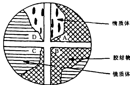
d) 边界情况——无效点
