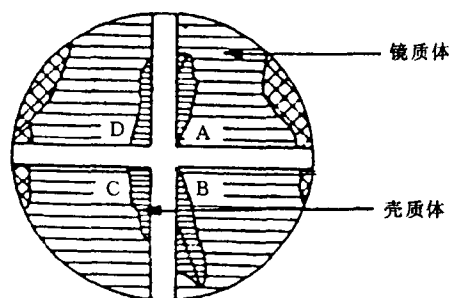
c) 边界情况——计数点 C(壳质体)
