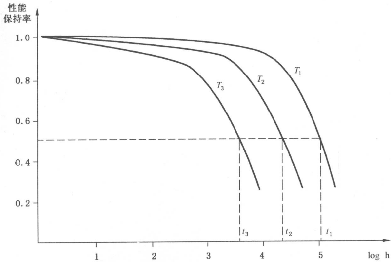
图 1 材料性能与老化时间
