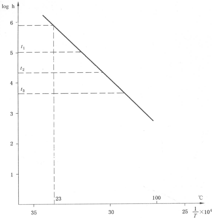
图 2 阿累尼乌斯图(时间-温度)
