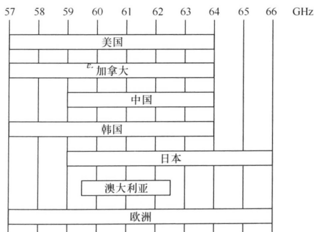
图 1-3 部分国家地区 60GHz 附近频段的规划
