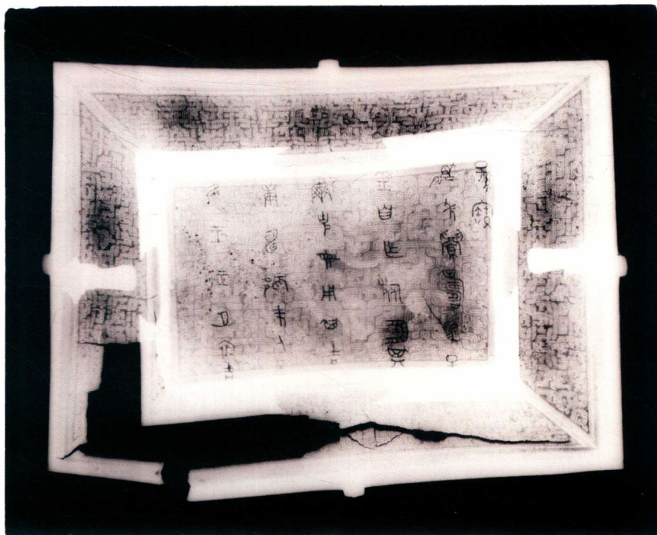
京山苏家垄墓地 M88 出土“胄夫人半克”簋及铭文 X 光片
