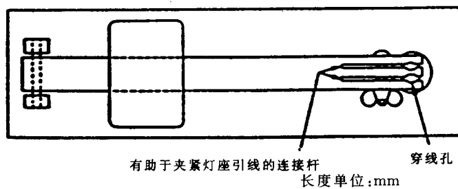
图 2 检验灯座连接安全性的试验装置
