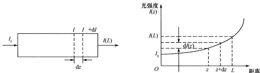
图 1-5 增益介质中的光放大
