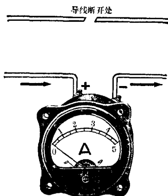
图 1-10 测量电流时电表的接法
