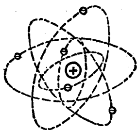
图1-1 电子围绕原子核旋转的情况
