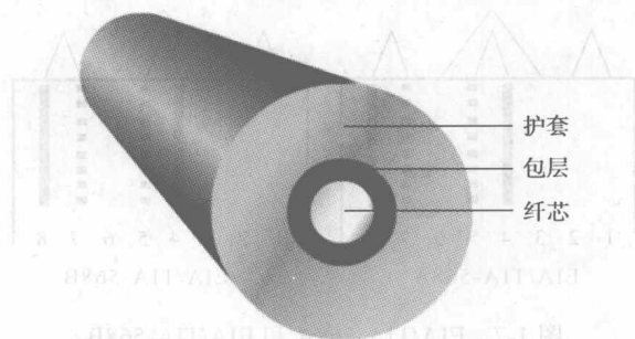
图 1-10 光纤的组成结构
