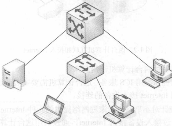
图 1-3 树型拓扑
