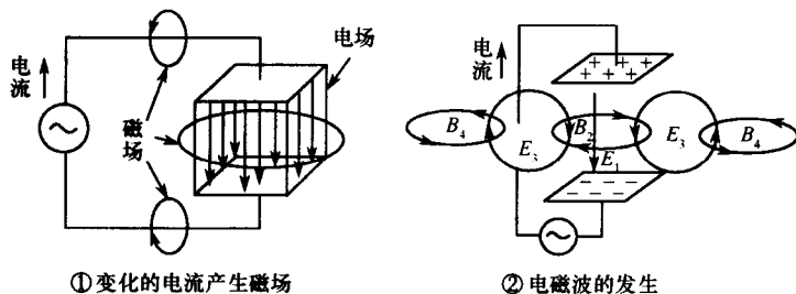
图 2-5 电磁波产生原理示意图
