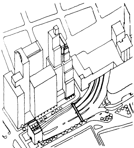
沿街高层建筑沿层高阶梯形后退也是解决天空暴露面矛盾的方法 (美) 纽约交易所大楼 (方案)
