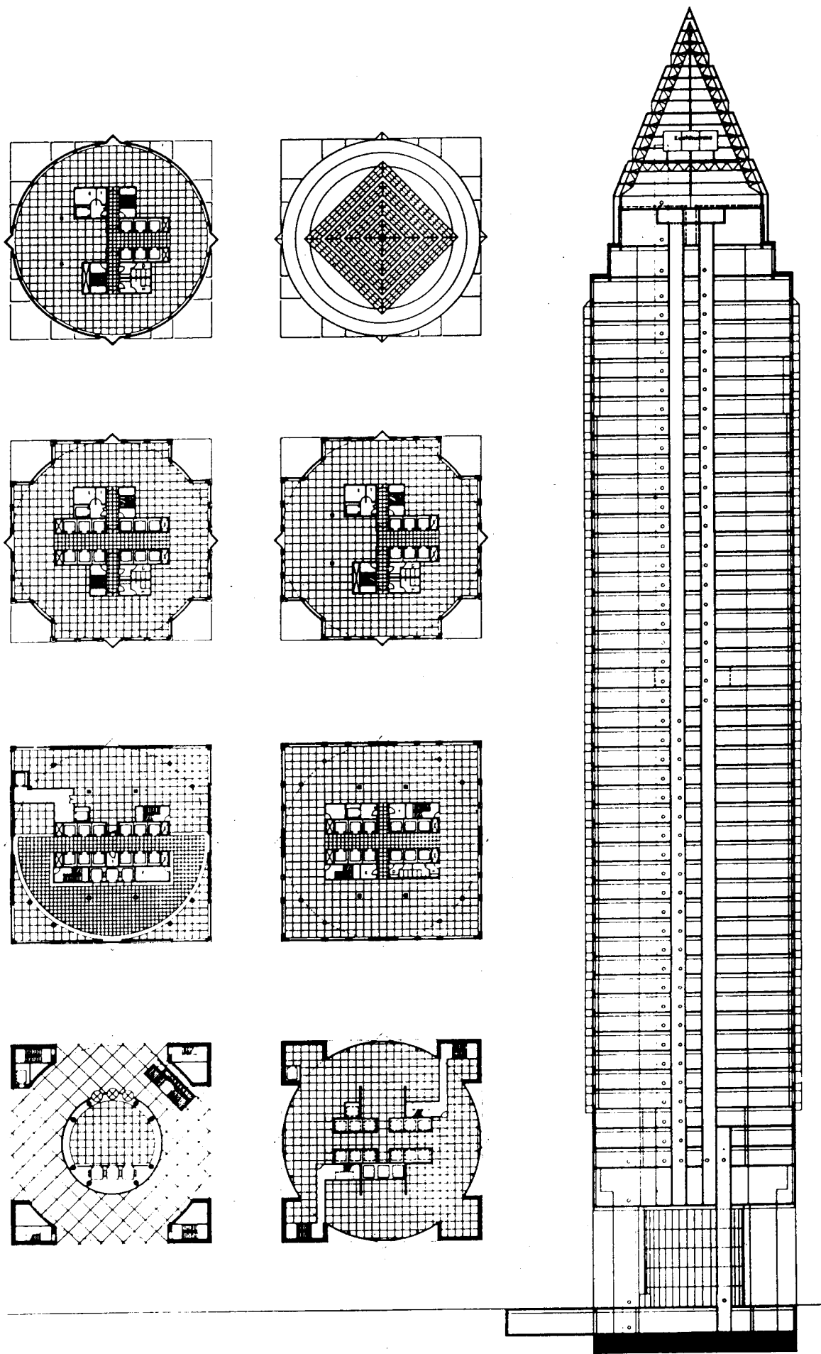
剖面
