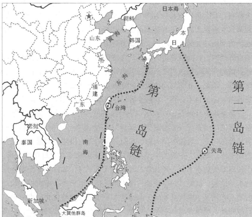
图 1-1 第一岛链和第二岛链示意图
