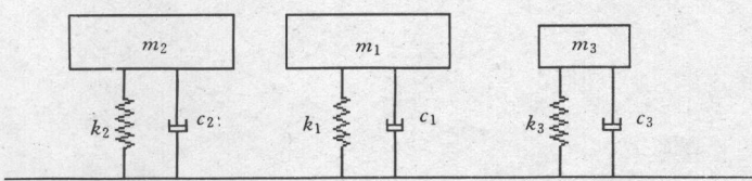
图 6 卧姿人体的模型
