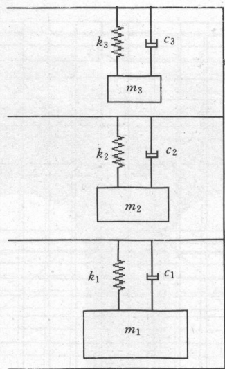
图 4 坐姿人体的模型
