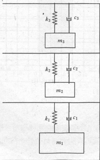
图 5 立姿人体的模型
