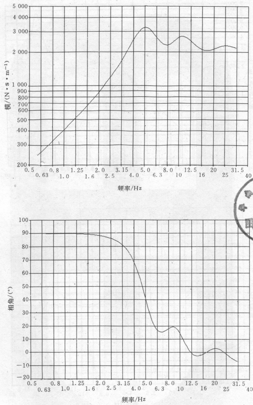
图 1 坐姿人体的机械驱动点阻抗 (根据 60 名受试者实测阻抗特性平均曲线拟合而成)
