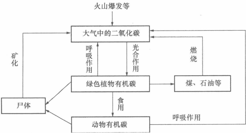
图 1-3 碳循环
