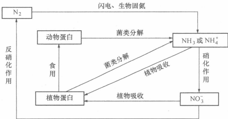
图 1-4 氮的循环图
