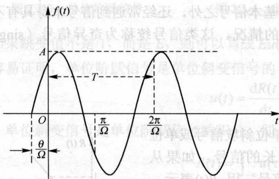
图 2.2-3 正弦信号
