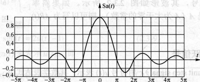
图 2.2-5 抽样函数
