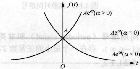
图 2.2-1 指数信号
