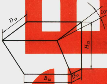
图 13 附接控制台的柜式和框架式仪表盘安装尺寸
