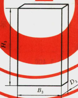
图 3 屏式仪表盘基本尺寸示意图
