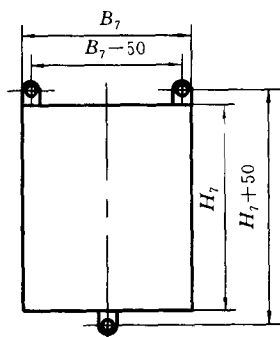
图 24 挂式仪表箱安装尺寸
