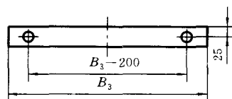
图 15 屏式仪表盘安装尺寸
