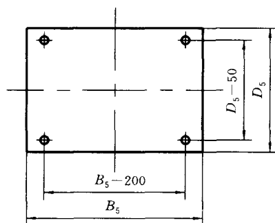
图 20 控制柜安装尺寸
