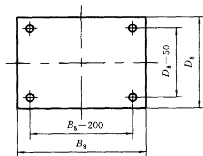
图 25 立式仪表箱安装尺寸
