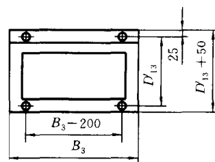
图 17 带附接控制台的屏式仪表盘安装尺寸
