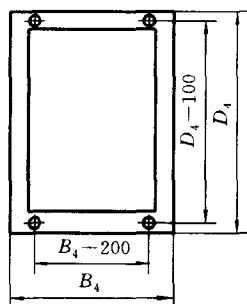
图 18 通道式仪表盘安装尺寸
