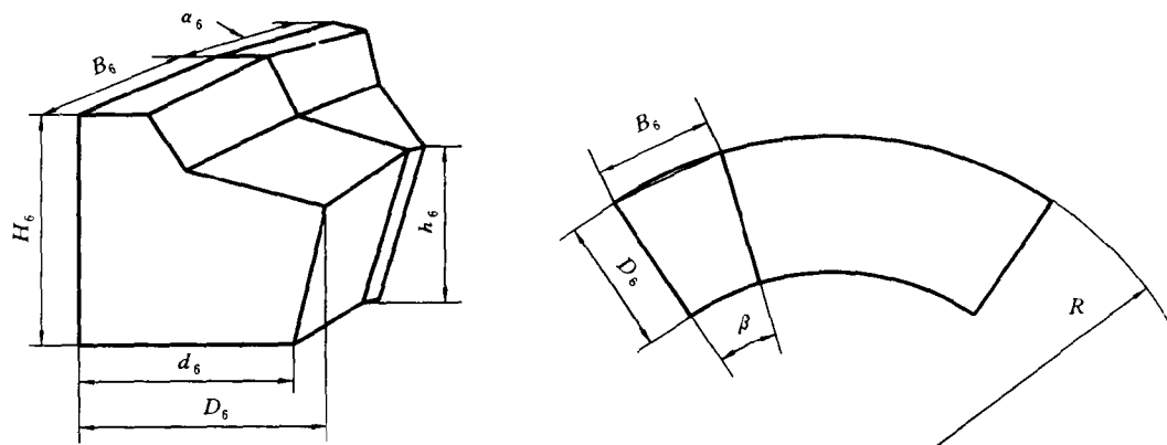
图 6 控制台基本尺寸示意图
