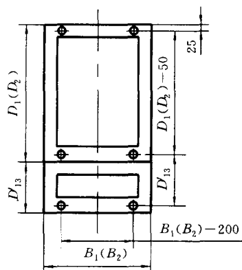
图 16 带附接控制台的柜式和框架式仪表盘安装尺寸
