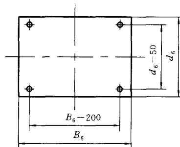
图 21 柜式和显示式控制台安装尺寸
