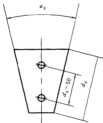
图 22 柜式和显示式弯连控制台安装尺寸
