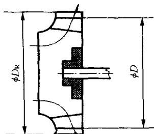
图 1 离心式风机的叶轮
