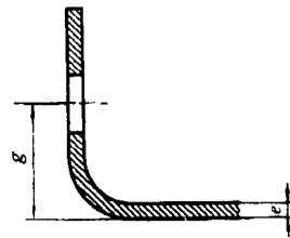
滚压式法兰设计
