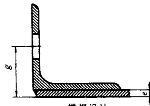
搭焊设计
