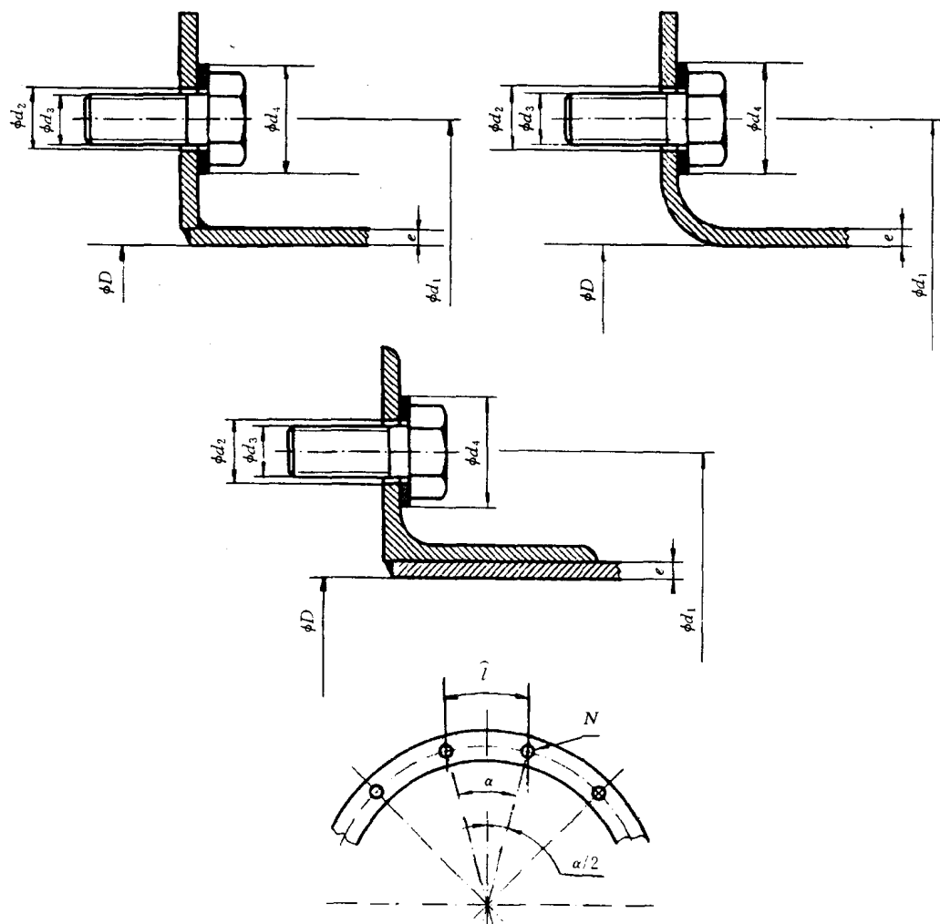
图 4 圆形法兰
