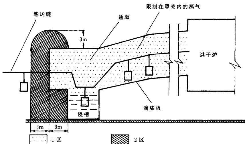
图 A2 封闭浸涂作业的爆炸危险区域划分图
