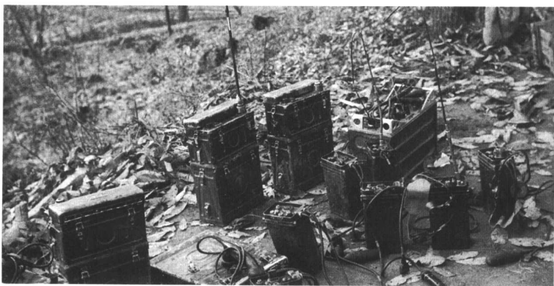
我军缴获英军的步话机。
