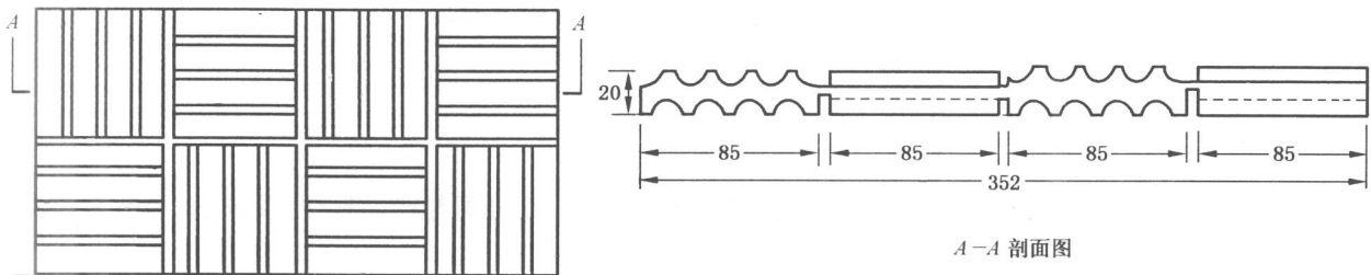
图 1 橡胶隔振垫产品结构
