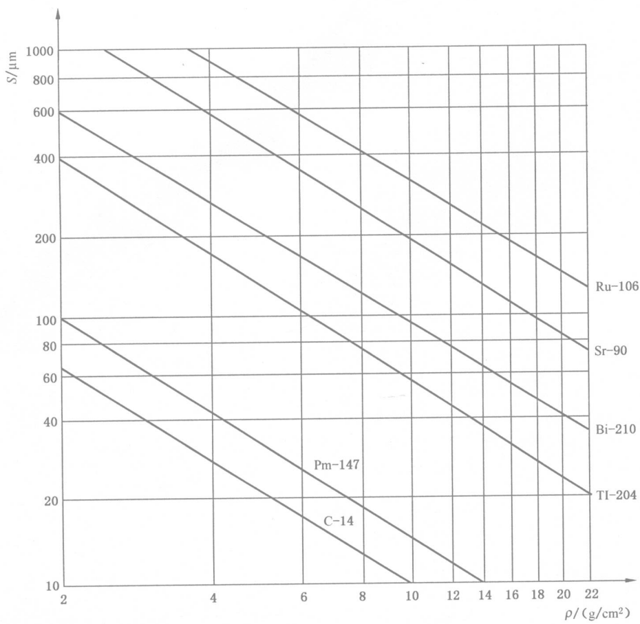
图 A.1 不同同位素饱和厚度 S 与密度 \rho 的关系
