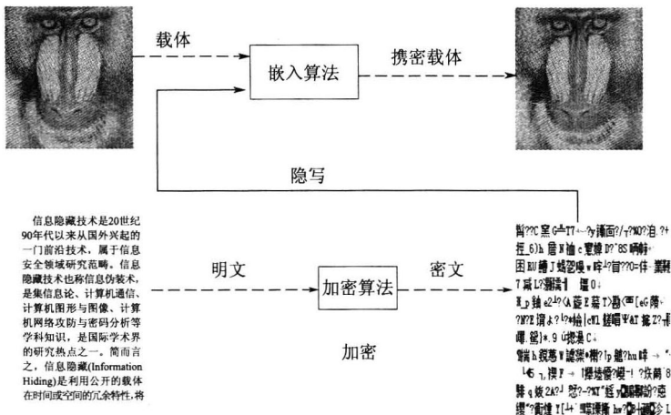
图 1-4 现代隐写术的基本原理
