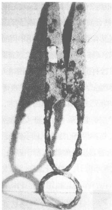
◎ 陕西宝鸡出土的交股式西汉铁剪
