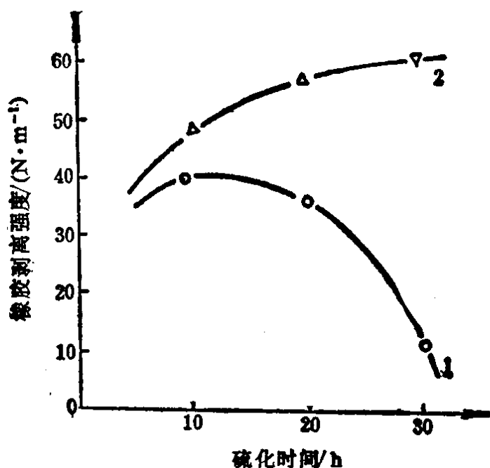
图1-4 硫化对橡胶胶接强度的影响
