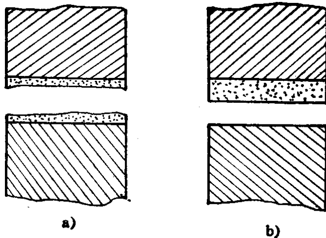
图1-3 胶接接头破坏的形式
