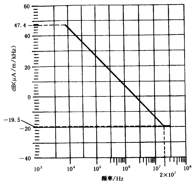
图 1 标准峰值脉冲的磁场强度推荐限值
