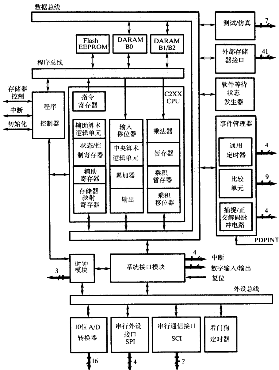
图 1-3 TMS320C24X 功能框图
