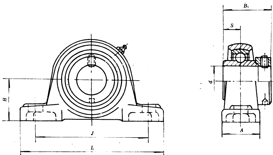
图 2 UELP 型
