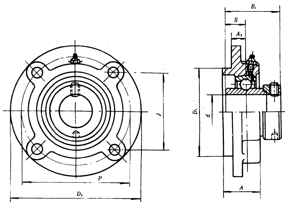
图 11 UELFC 型
