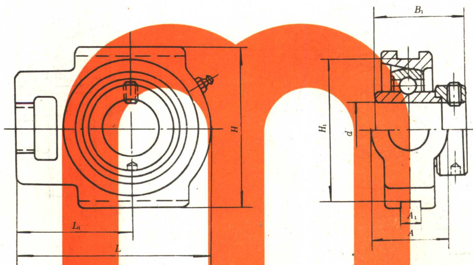
图 14 UELK 型
