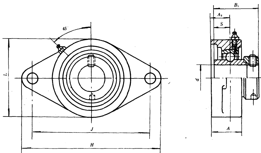
图 8 UELFLU 型
