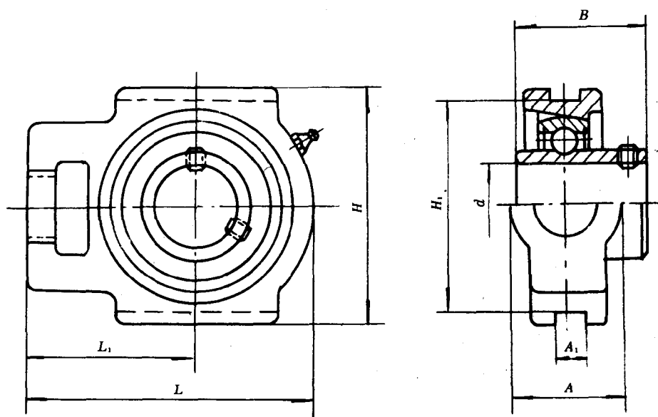
图 13 UCK 型
