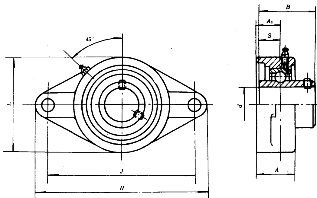
图 7 UCFLU 型
