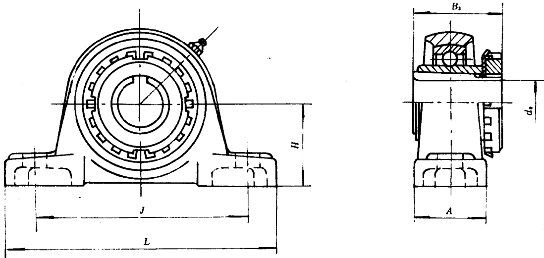
图 3 UKP+H 型
