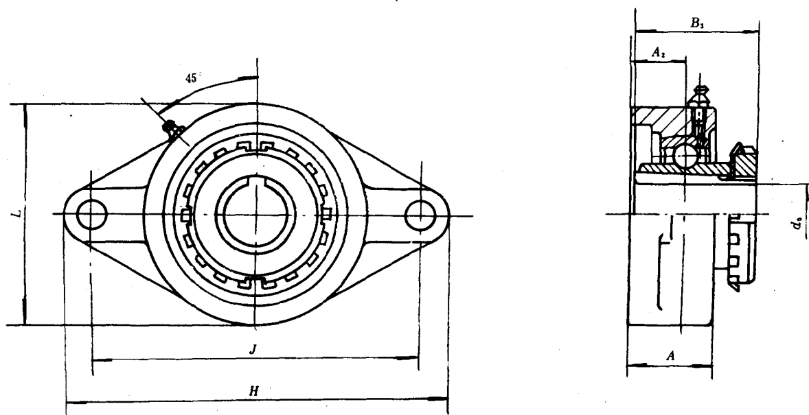
图 9 UKFLU+H 型
