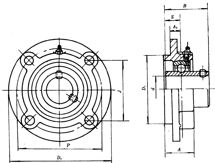
图 10 UCFC 型
