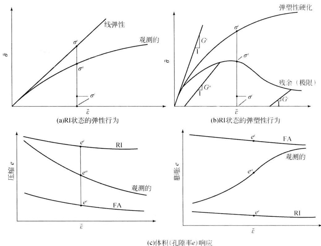
图 1.3 不同材料行为的扰动示意图
