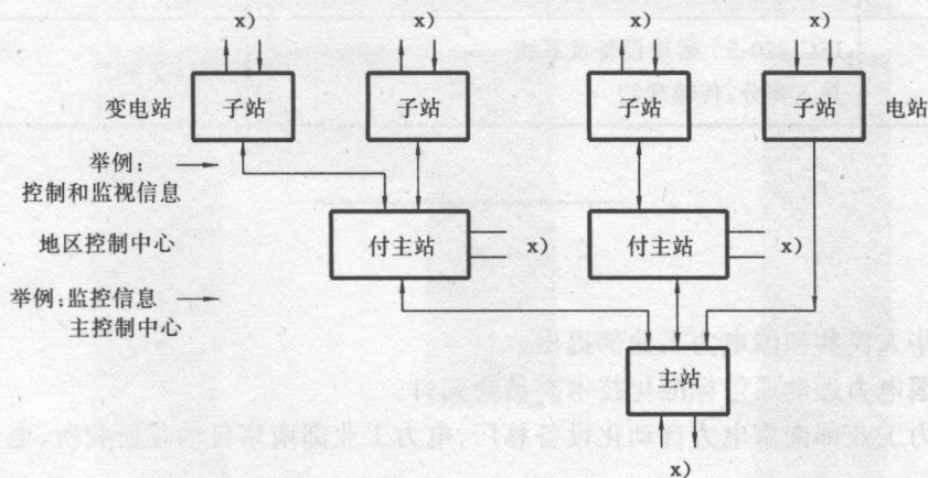
图 1 数据流的方框图(举例)
