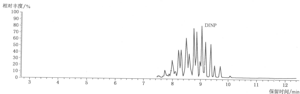
图 C.4 DINP 标准物的 GC-MS 选择离子( m/Z=293 )色谱图
