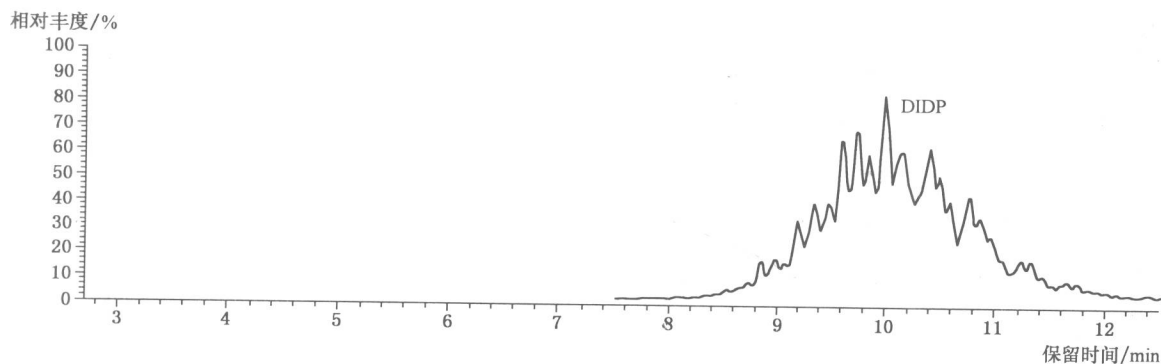
图 C.5 DIDP 标准物的 GC-MS 选择离子( m/Z=307 )色谱图
