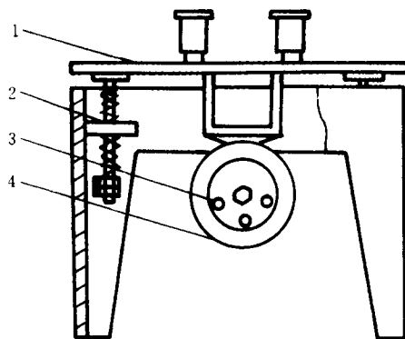
1—台板;2—弹簧;3—偏重轮;4—电机
