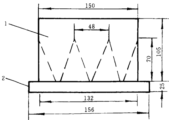
1—漏斗;2—模套
