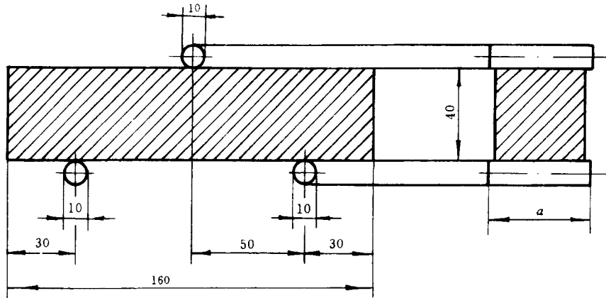
图 5 抗折强度测定加荷图
