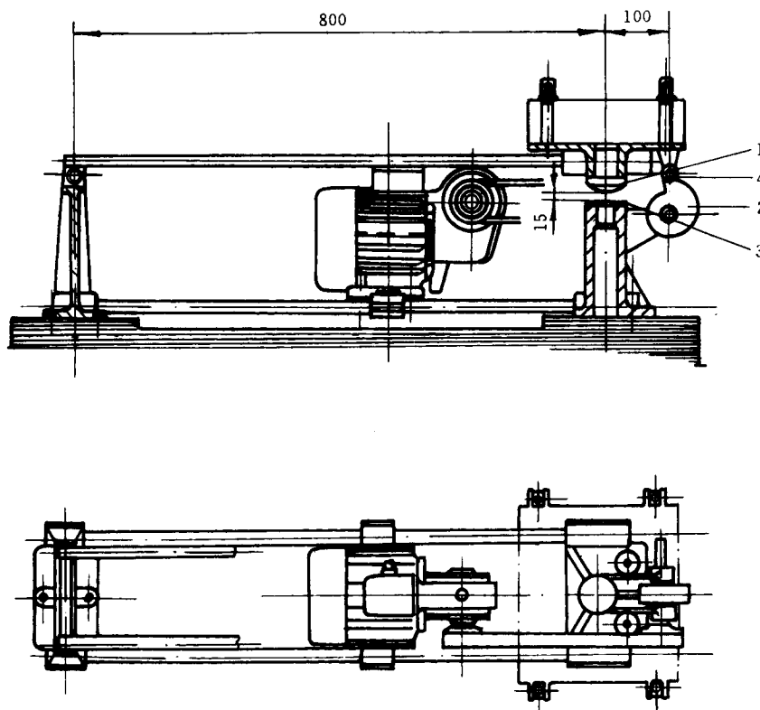
1—突头; 2—凸轮; 3—止动器; 4—随动轮
