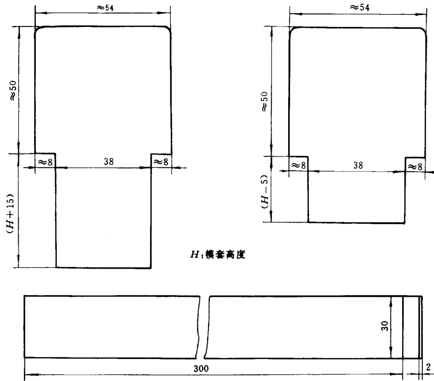
图 3 典型的播料器和金属刮平尺
