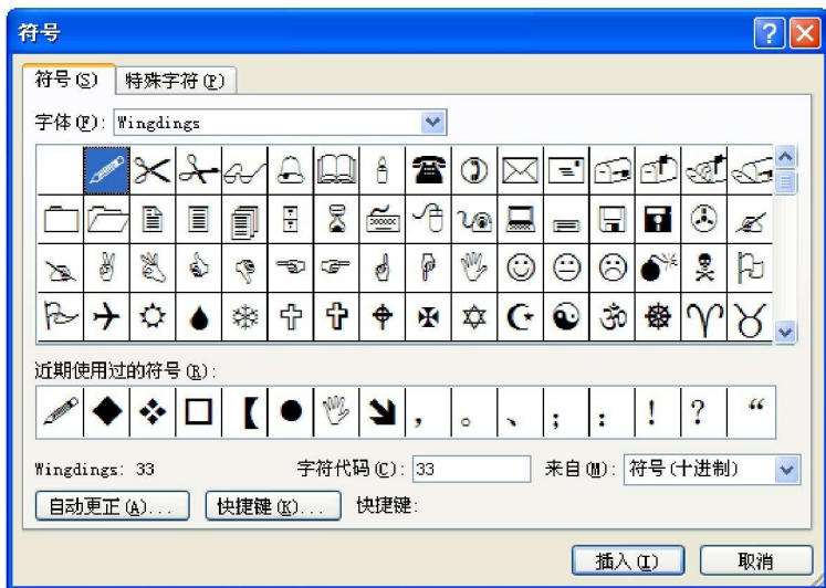
图 1-9 “符号”对话框
