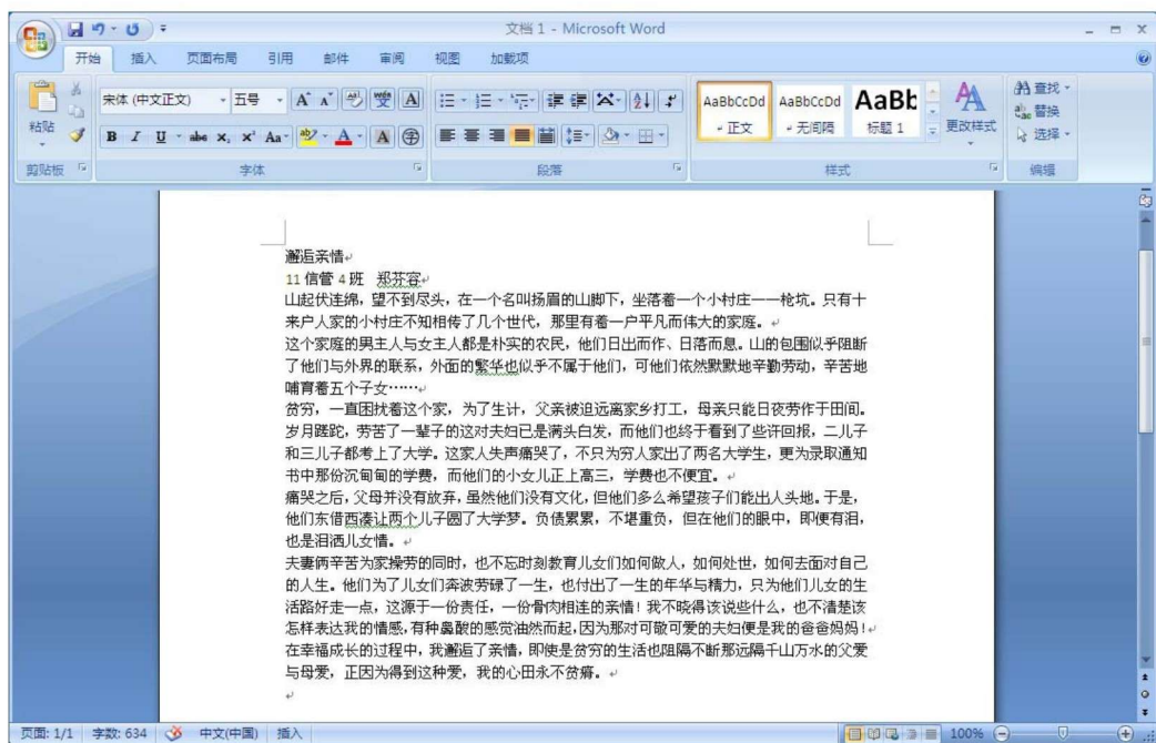
图 1-8 输入文本
