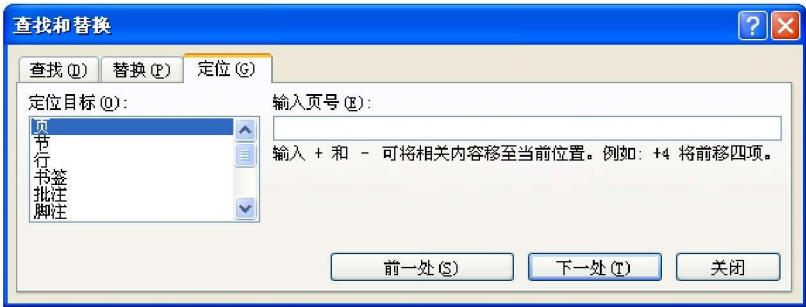
图 1-12 “定位”选项卡
