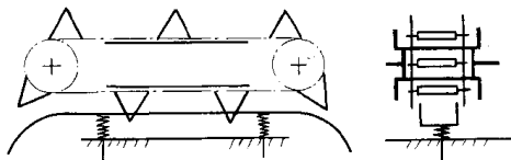
(16) 夹持式禾秆输送机
