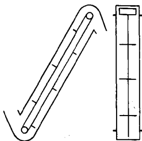
(16) 夹持式禾秆输送机
