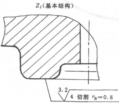
图 2 密封表面和连接螺纹的尺寸
