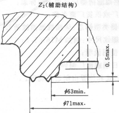
图 2 密封表面和连接螺纹的尺寸
