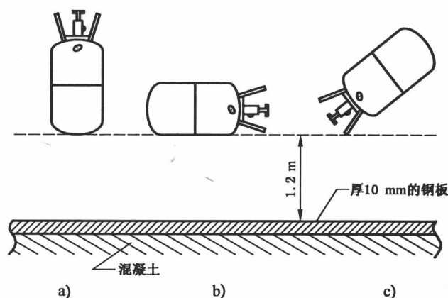
图 A.2 跌落试验
