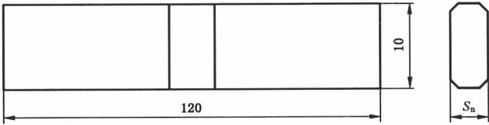
图 B.3 弯曲试样
