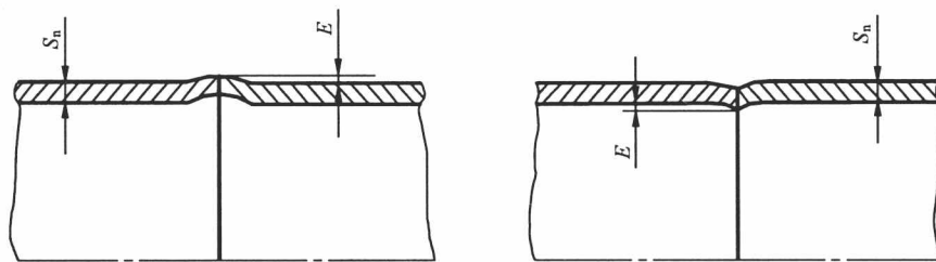
图2 环焊缝棱角高度
