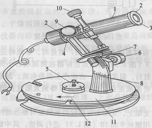
图 1.3 直接辐射表
