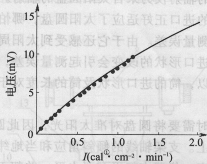
图 1.2 辐射表的输出电压与入射光辐射通量密度
