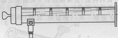
图 1.4 直接辐射表的进光筒
