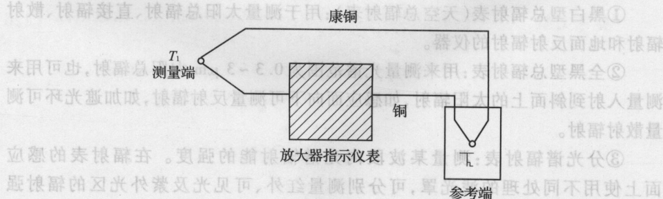
图 1.1 热电偶测温电路
