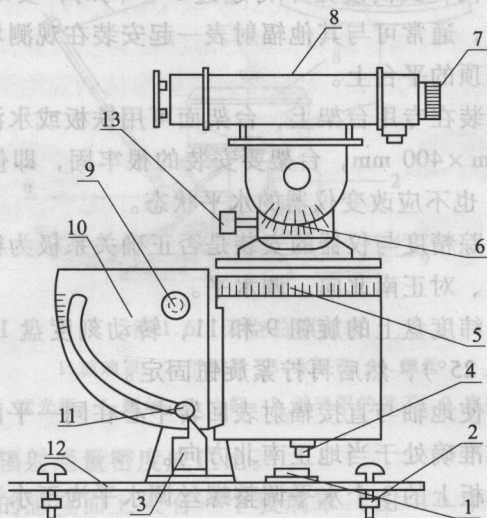
图 1.5 TBS—2—B 直接辐射表
