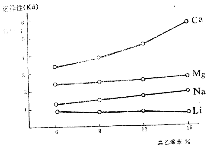
图1.3 不同含量二乙烯苯交联的阳离子交换剂的选择性(聚苯乙烯磺酸树脂)
