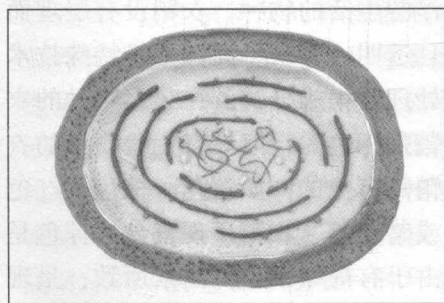
蓝藻模型图
