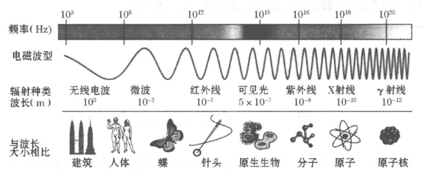
图 1-1 电磁辐射谱
